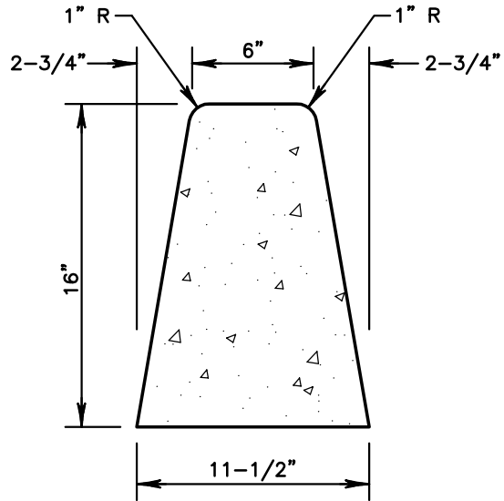
TYPE E-4 CURB
