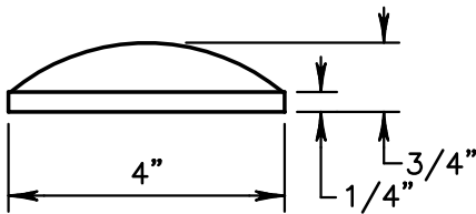
RUMBLE BAR
